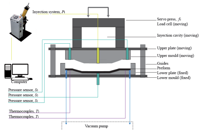
Figura 1: Esquema del molde.
