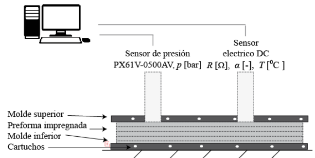
Figura 3: Esquema de la caracterización del sensor.
