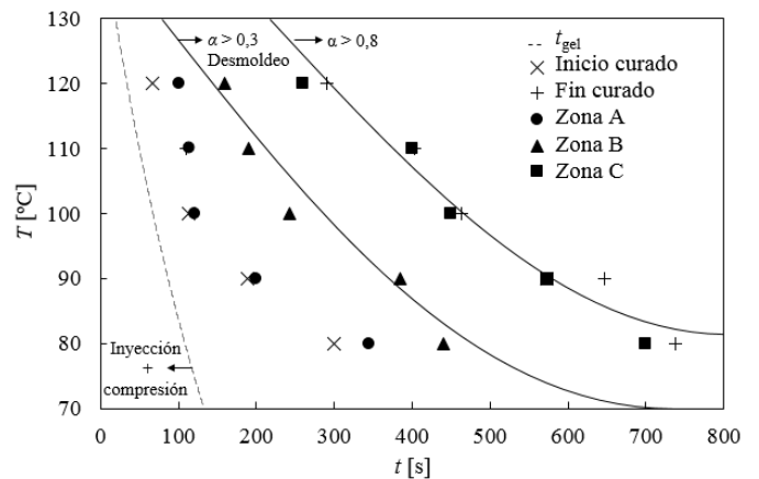
Figura 5: Ventana de procesos que relaciona la temperatura de curado con los tiempos de cada etapa.
