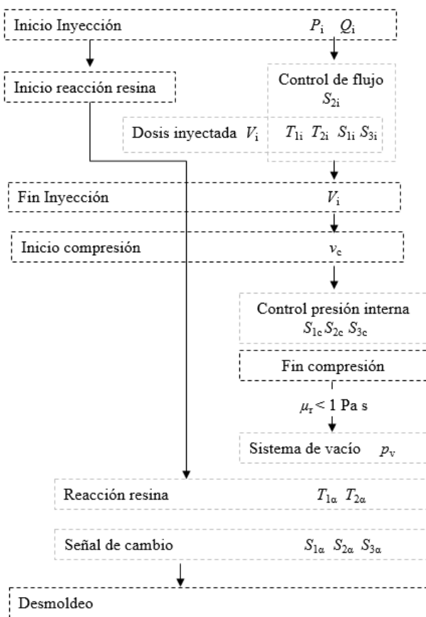
Figura 2: Diagrama de control de flujo.
