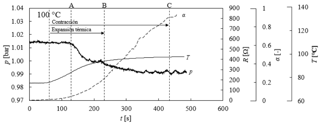
Figura 4: Señal de los sensores.
