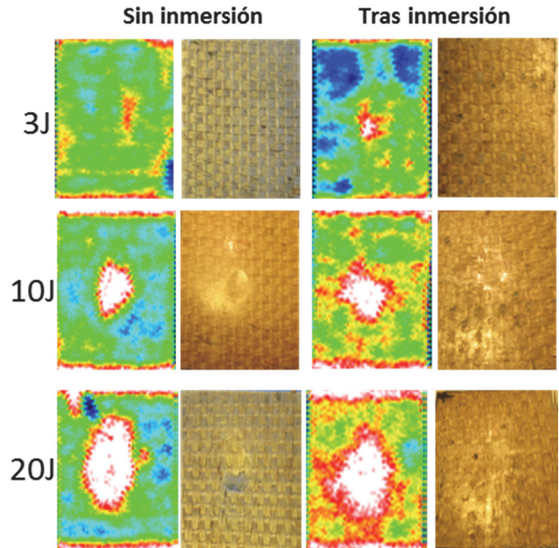
Figura 8. Imágenes de C-Scan de zonas de impacto de material sin inmersión y tras inmersión en agua de mar. Fuente: Los autores
