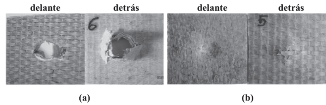
Figura 7. Probetas de biocomposite reforzado con fibra de Figue sin inmersión (a) y tras inmersión en agua de mar (b) a energía de impacto E_0=25J . Fuente: Los autores
