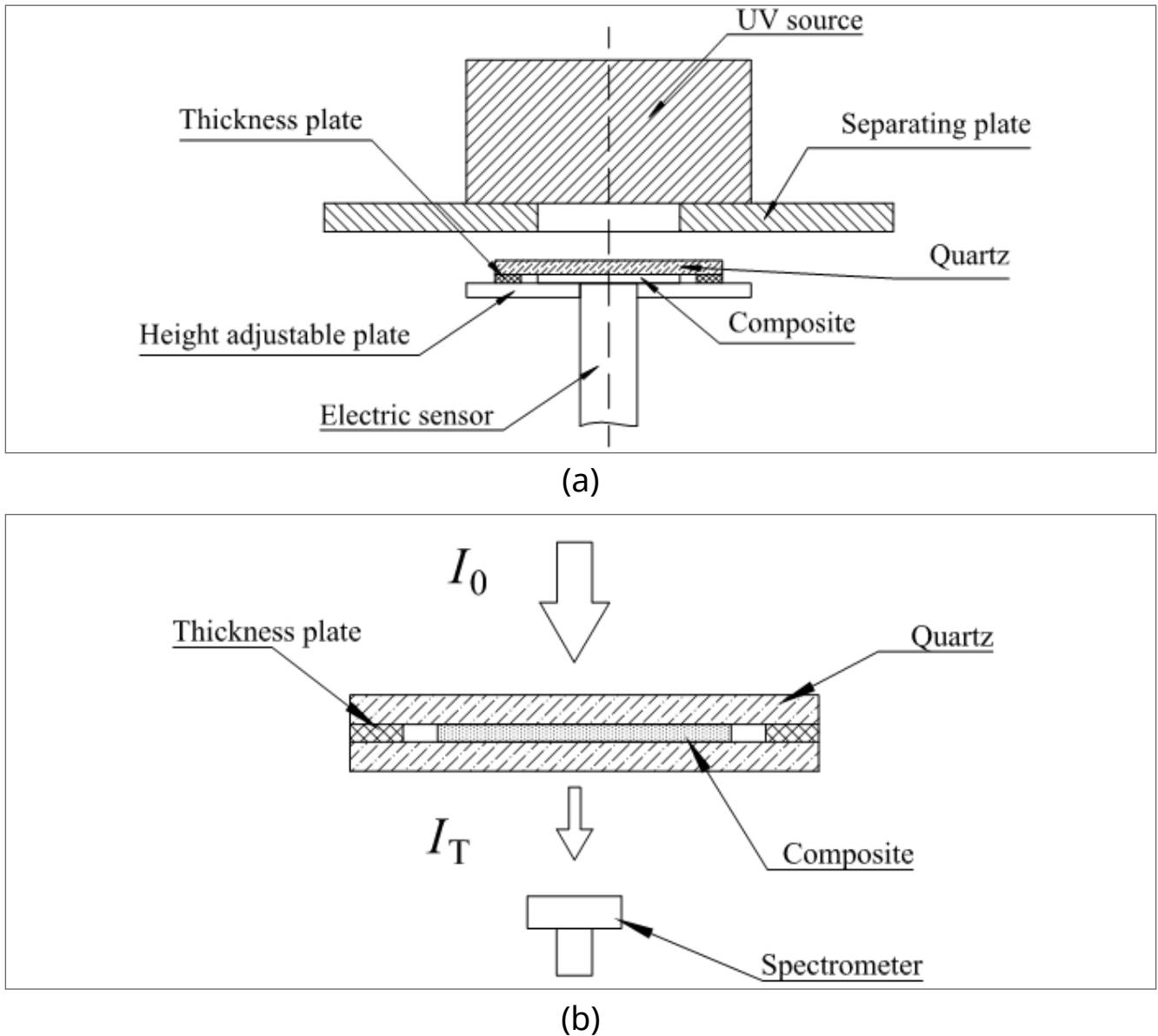
Figura 1. Diagramas de los utillajes de análisis del curado (a) y del análisis óptico (b).
