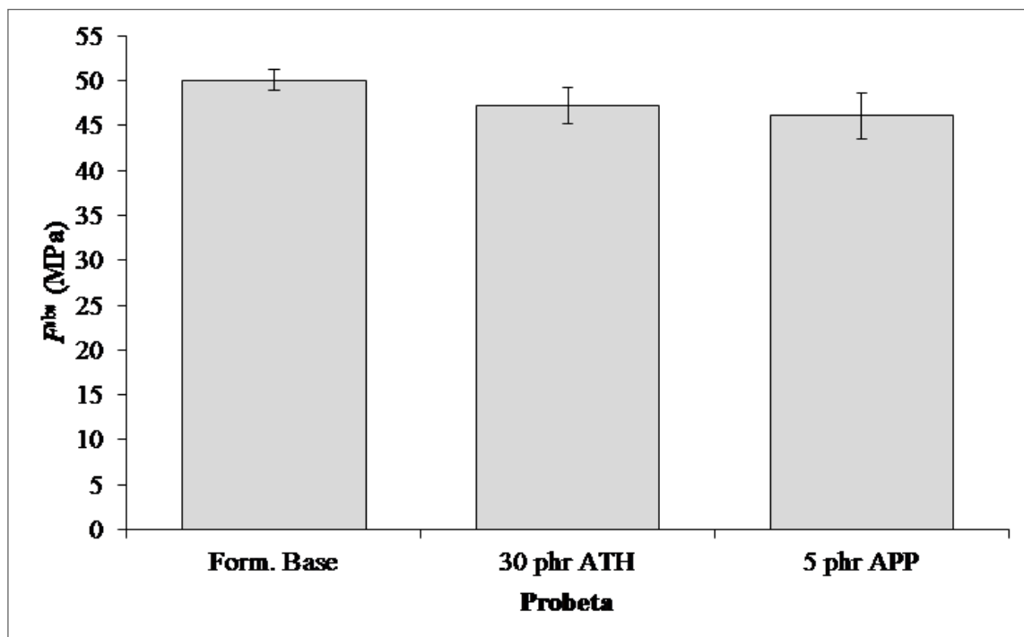
Figura 6. Valores de ILSS para las diferentes formulaciones analizadas.
